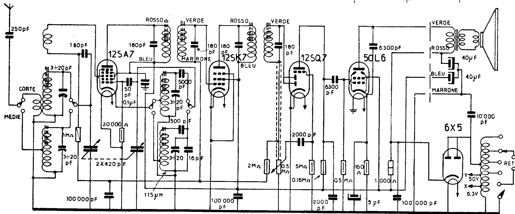
DUCATI SSR - Modd. RR 2050, RR 2051 e RF 2055 - Medie da 580 a 185 m, corte da 55 a 18,7 m. Media frequenza a 462 kc per i RR ed a 468 kc per il RF. Uscita 1,4 W. Consumo 45 W. Finale: placca 140 V, schermo 115 V e catodo 7 V. Conv. e ampl. MF.: placche e schermi 115 V.
